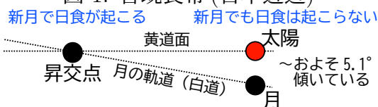
図 2: 日食の条件
