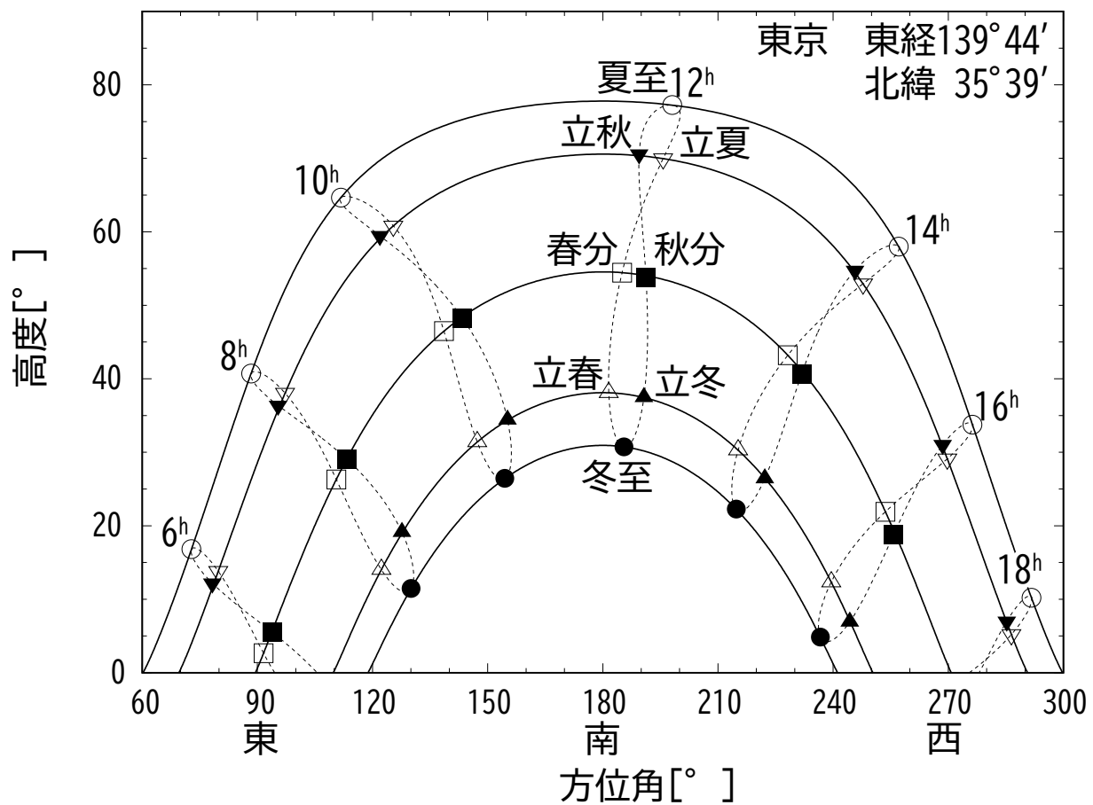
図は東京における1年間の太陽の高度と方位角。 記号は●：冬至，△：立春，□：春分，▽：立夏， ○：夏至，▼：立秋，■：秋分，▲：立冬を表す。
