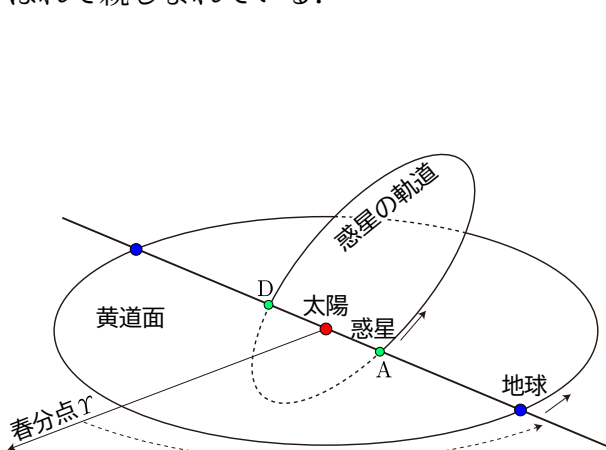
図1: 惑星の軌道
